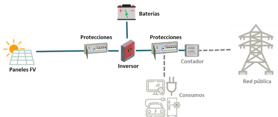
FIGURA 2.1 Partes de una instalación fotovoltaica de autoconsumo
